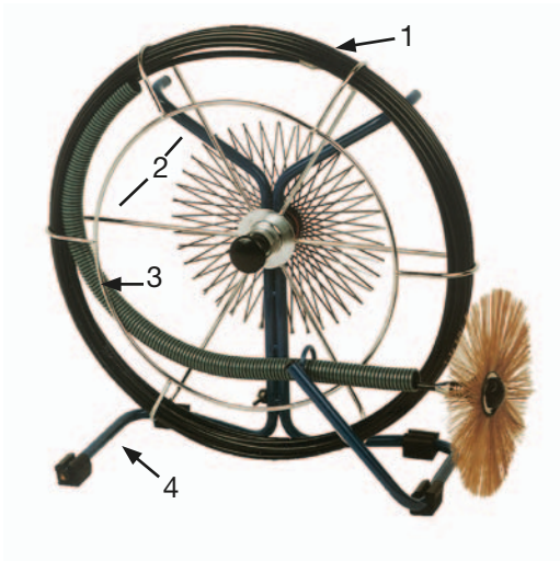
Figuur 2.1: Wöhler veegstanghaspel
