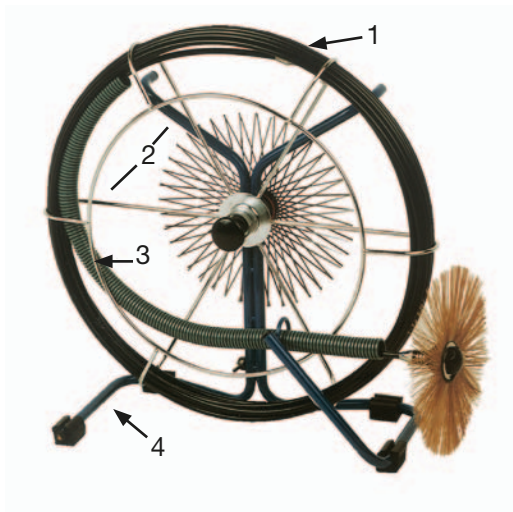
Abbildung 2.1: Aufbau der Kehrstangenhaspel
